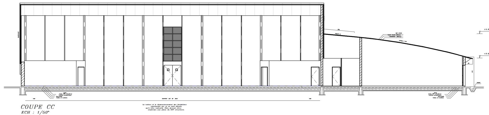
Coupe 1 1 : 200
